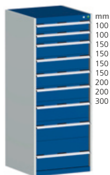
Šírka 650
